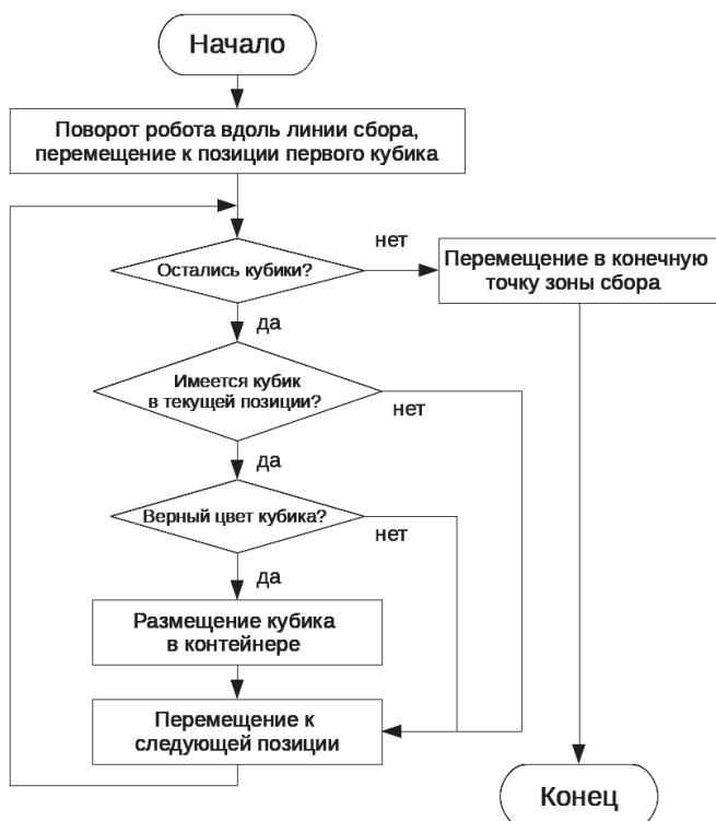
Рис. 5. Алгоритм сбора кубиков
