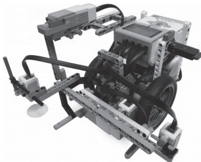
Рис. 6. Робот-ткач: вид сбоку
