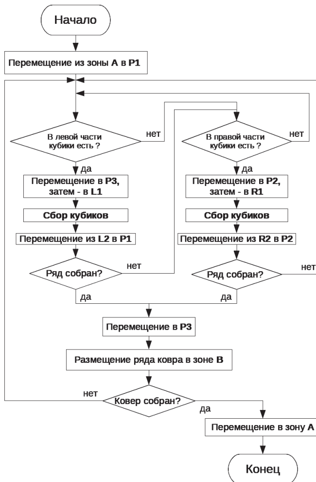
Рис. 4. Общий алгоритм решения задачи
